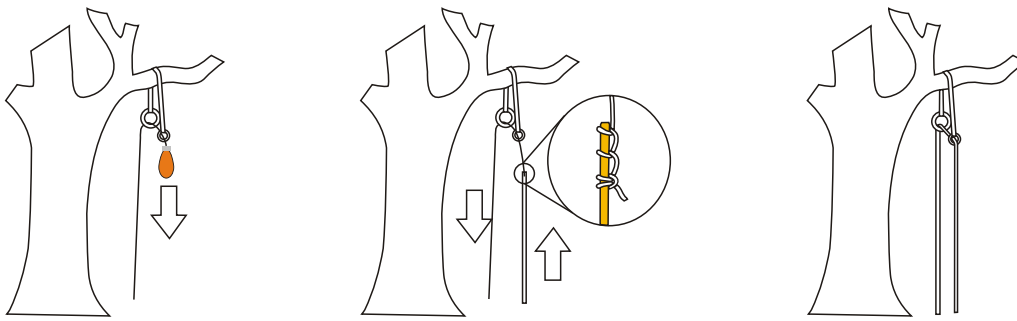
Benutzung des Wurfbeutels TREEMOUSE zur Installation eines JINGLE Cambiumschoners im Baum.
